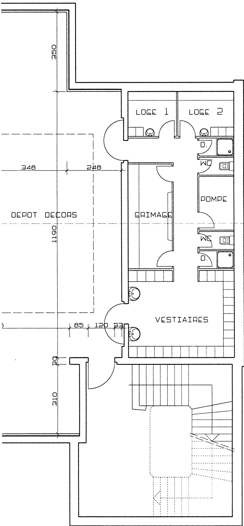
PLAN DE SCENE / ECH.: 1-100 / 12090
